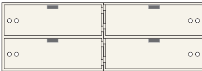
AXL-4-10 (Wt. 145 lbs.) 4 openings ea. 5" x 16"
